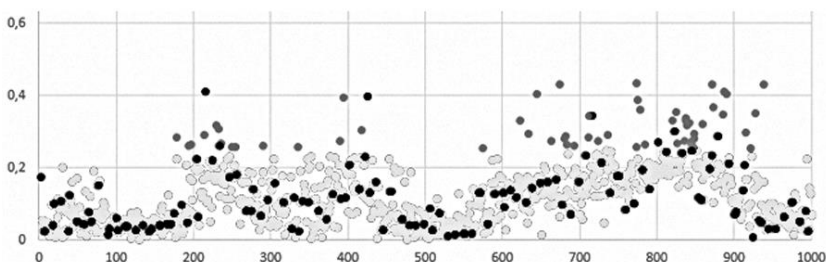
Рис. 2. Пример выполнения одной криволинейной траектории. По горизонтальной оси – итерации измерений. Вертикальная ось – ошибка локализации. Светло-серые точки – «хорошая», серые – «плохая» локализация. Черные точки – случаи, когда алгоритм нашел положение робота, но признал локализацию неопределенной.
