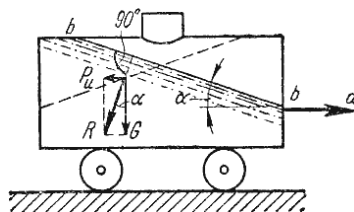
Рис. 4. 2. Относительный покой жидкости при прямолинейном движении сосуда
