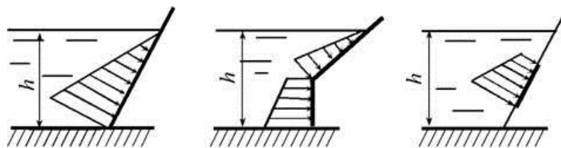
Рис. 2. 4. Эпюры давления
