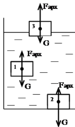
Рис. 4. 7. Закон Архимеда
