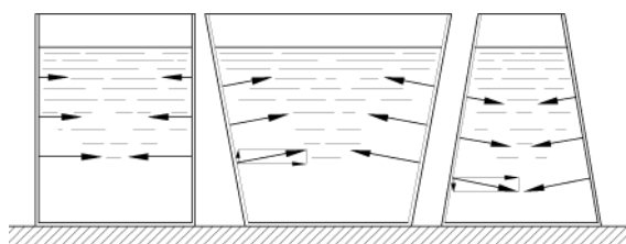
Рис. 4. 5. Гидростатический парадокс
