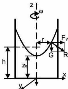
Рис. 4. 3. Относительный покой жидкости в цилиндрической емкости На
