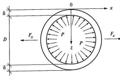
Рис. 4. 8. К определению толщины стенки
