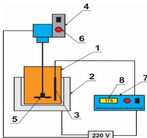
Рис. 2. Схема установки модификации битума
