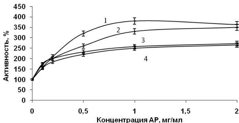
Рис. 1. Влияние окисленных АР на каталитические активности ферментного препарата «Полифермент»: 1 - протеолитическую (t=37С, рН=8.0-8.2), 2 - амилолитическую (t=30С, рН=7.0), 3 - целлюлазную ( t=50С, рН=4.7), 4 - ксиланазную ( t=50С, рН=5.0)
