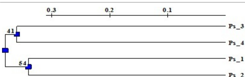
Рис. 1. UPGMA-дендрограмма генетического сходства популяций P. sylvestris , построенная на основании полиморфизма ISSR-маркеров. Шкала сверху - генетические дистанции по Ней и Ли [8]. На дендрограмме цифрами указаны значения бутстрепа (в %).
