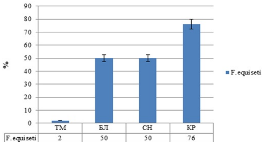
Рис. 1. Рост Fuzarium equiseti при разных спектрах света (7 сутки)
