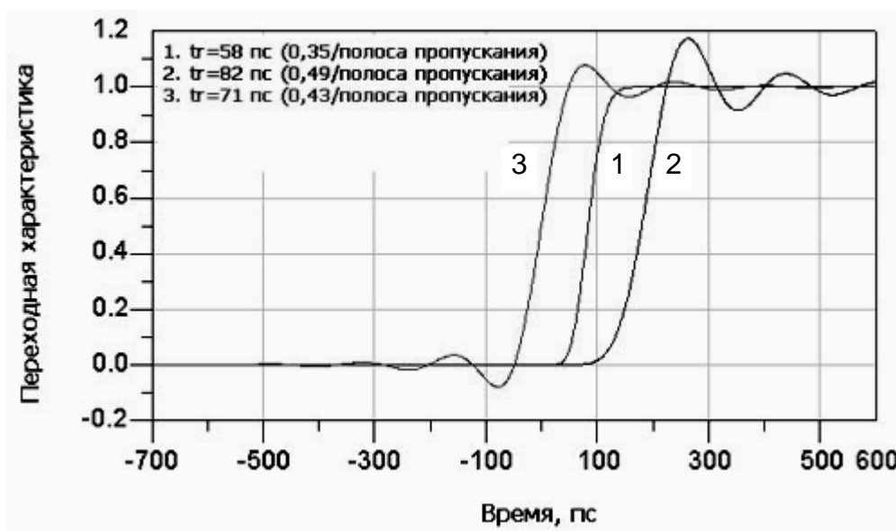
Рис. 2.7. Переходные характеристики осциллографов с гауссовой АЧХ (1), с максимально плоской АЧХ (2) и с АЧХ Бесселя (3) фазовой характеристики (АЧХ Бесселя) (3).
