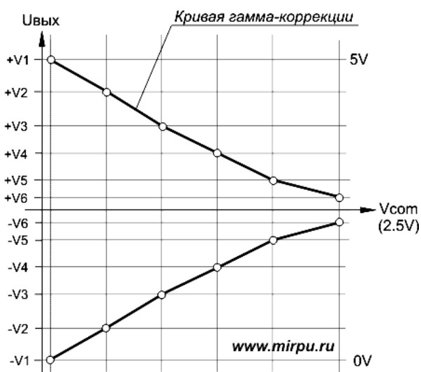
Рис. 2.21. Кривая гамма-коррекции
