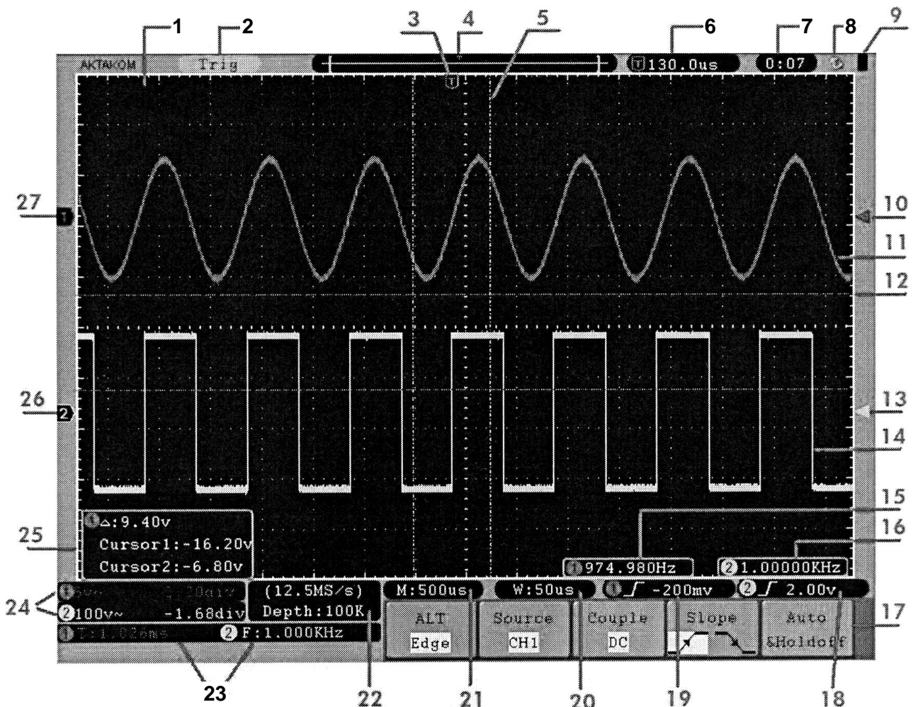
Рис. 3.3. Дисплей осциллографа
