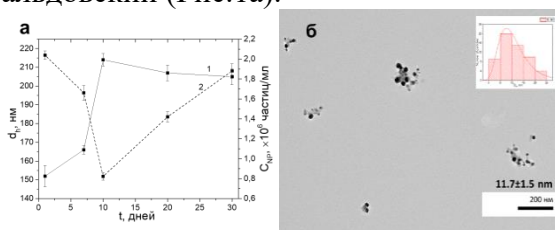
Рисунок 1 – Зависимость изменения среднего значения гидродинамического диаметра (1) и концентрации (2) частиц AgNPs-4 ( n_{Ag^+}:n_{(NH(CH_2)_2NH_2)\text{-фрагменты}}=1:4 ) в водном растворе от времени (а) по данным НТА. Данные ПЭМ образца AgNPs-4 (б) и диаграмма распределения частиц.
