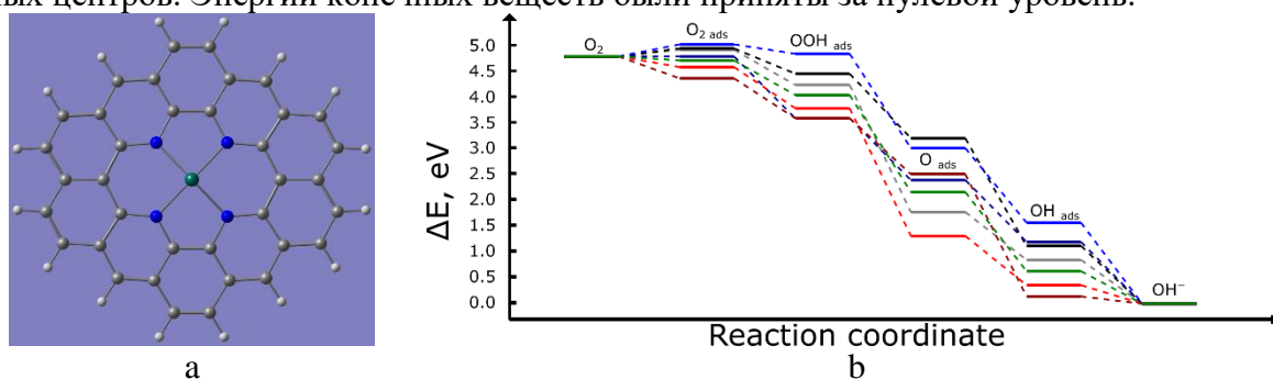
Рисунок 1 – Структура модельного катализатора. Серые сферы – углерод, синие – азот, белые – водород, зелёный – исследуемый металл (а); Энергетический профиль ORR на модельных катализаторах: CoN 4 -серый; CuN 4 -черный; NiN 4 -синий; MnN 4 -красный; ZnN 4 -темно-красный; Cr(OH)N 4 -зеленый. Идеальный катализатор - темно-синий (b).
