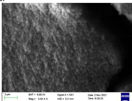
Рисунок 1 – Морфология марганецсодержащей поверхности стеклоуглерода.
