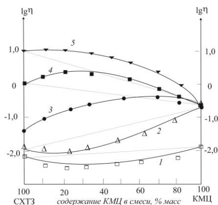
Рисунок 1 – Зависимость динамической вязкости, определенной при частоте осцилляции 0,1 Герц, от соотношения полимеров в смеси для растворов СХТЗ-КМЦ с концентрацией 0,5 г/дл-0,3 г/дл (1), 0,5 г/дл-0,5 г/дл (2), 1,0 г/дл-1,0 г/дл (3), 3,0 г/дл-1,0 г/дл (4), 5,0 г/дл-1,0 г/дл (5). Размерность исходной \eta – в Па*с.
