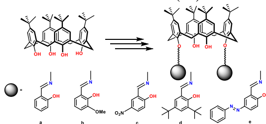
Рисунок 1 – Макроциклические основания Шиффа на основе дизамещённых производных (тиа)каликс[4]аренов с иминофенольными координирующими центрами.
