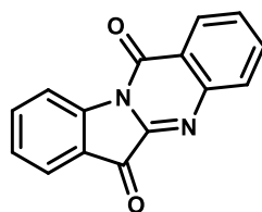
триптантрин
