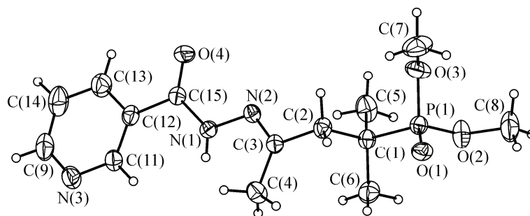
Рис. 2. Геометрия молекулы III ( E_{C=N}E_{N-N}Z_{N-C(O)} -изомер) в кристалле. Параметры тепловых колебаний приведены с вероятностью 30 %
