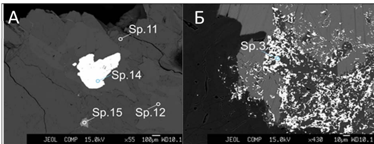
Рис.1. А- парагенезис тип 5(1). Sp-11 – alexandrite, Sp-12 – emerald, Sp-14 – monazite, Sp-15 – fluorite; Б- парагенезис тип 5(2). Sp-3 – allanite, light gray – floopite, mediumgray is emerald, dark gray is alexandrite.
