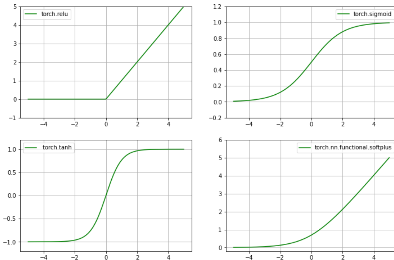
Рис.26 Графики функций активации (ReLU, sigmoid, tanh, softplus)
