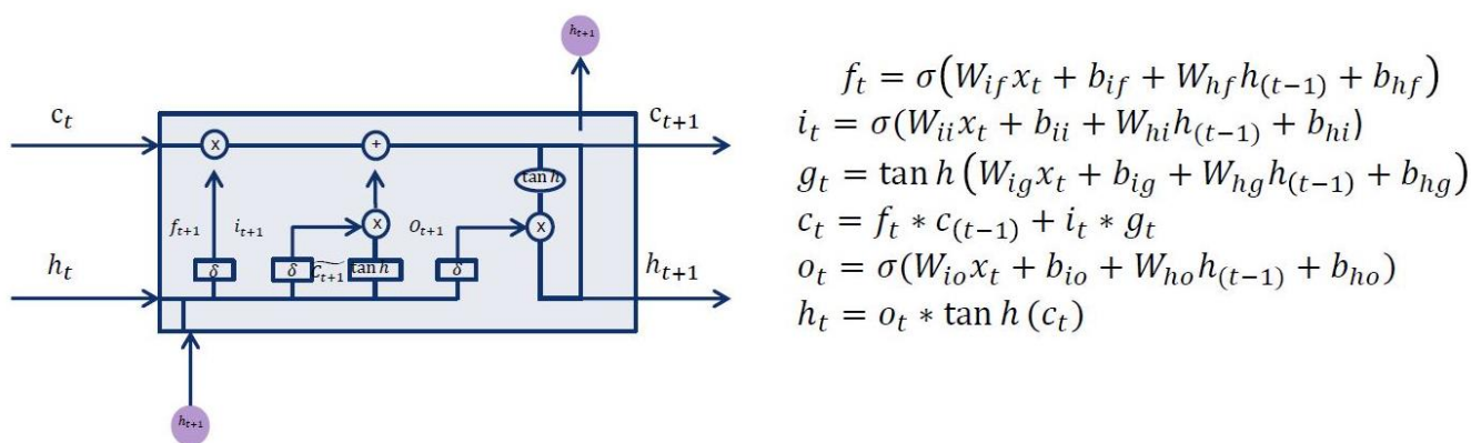
Рис. 51 Схематическое изображение LSTM ячейки
