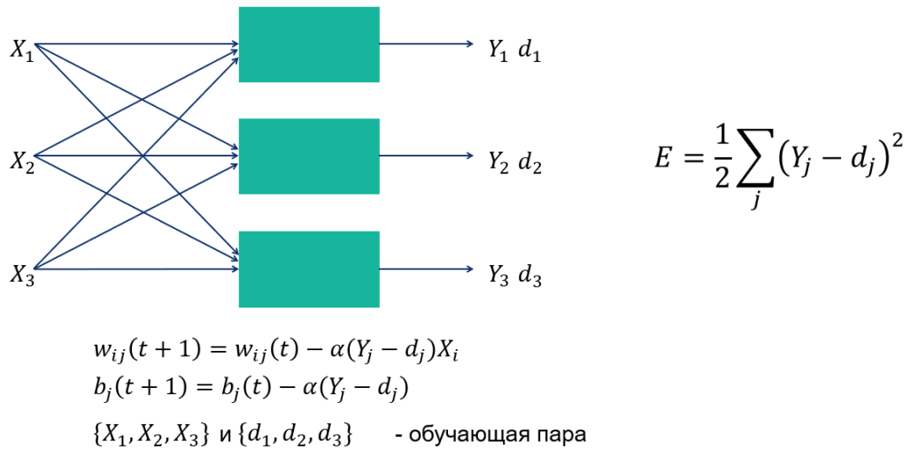
Рис.30 Обучение однослойной нейронной сети (алгоритм Уидроу-Хоффа)
