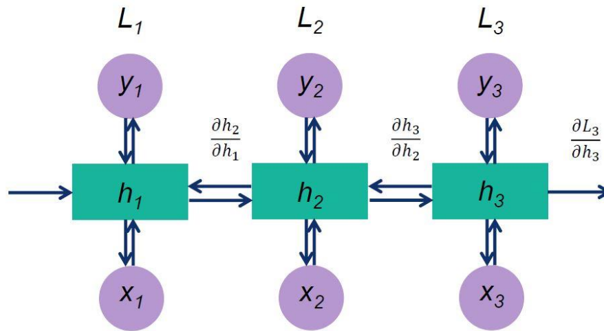
Рис. 49 Схема «алгоритма обратного распространения ошибки сквозь время»
