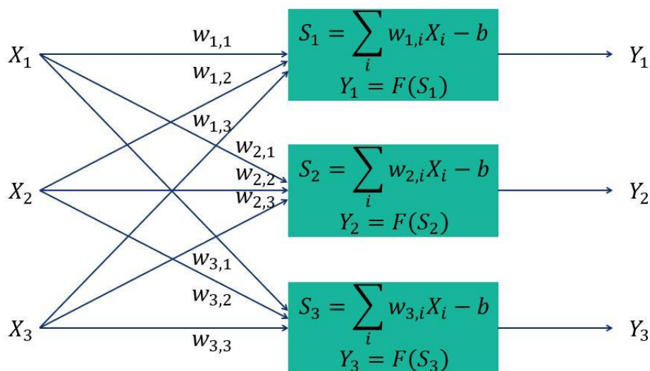
Рис.28 Однослойная нейронная сеть
