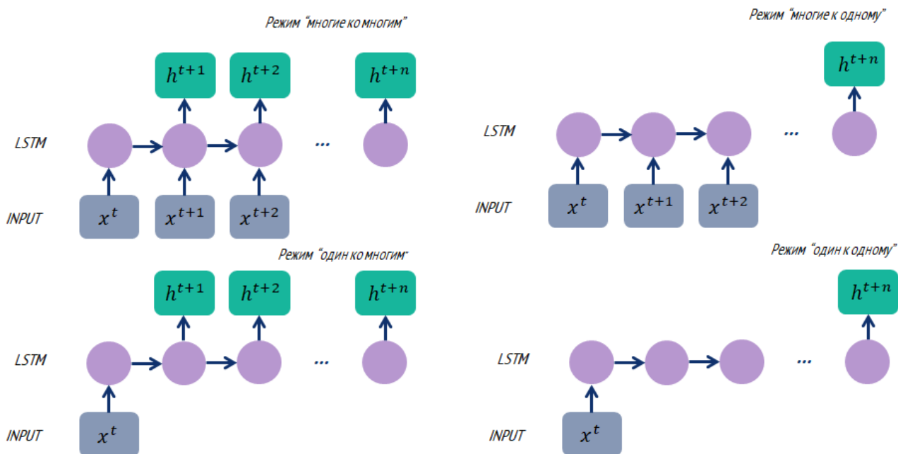
Рис. 53 Режимы работы рекуррентных нейронных сетей
