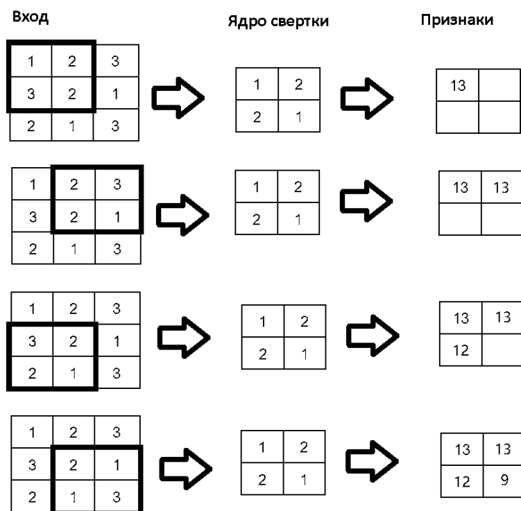
Рис. 68 Графическая изображения операций свёрточного слоя
