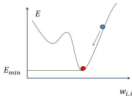
Рис.29 Метод градиентного спуска в пространстве весовых коэффициентов
