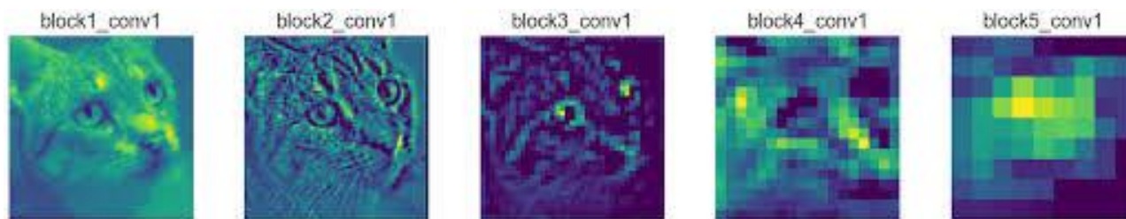
Рис. 72 Интерпретация работы свёрточной нейронной сети
