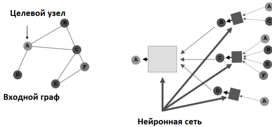
Рис. 82 Вычислительный граф
