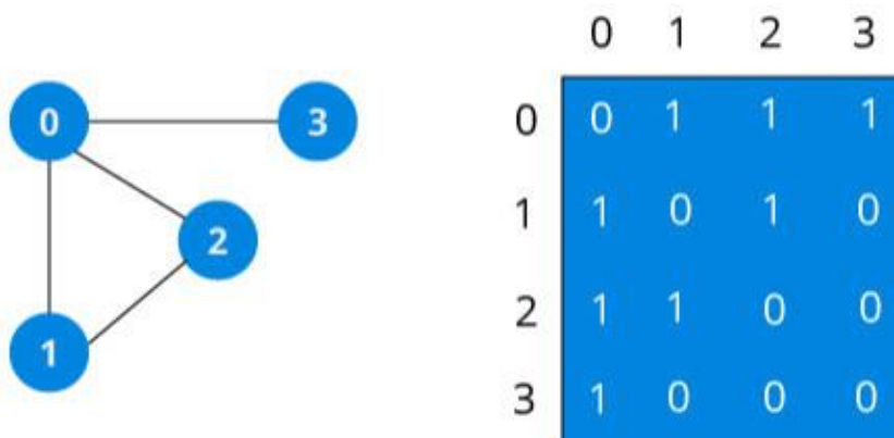
Рис. 78 Матрица смежности
