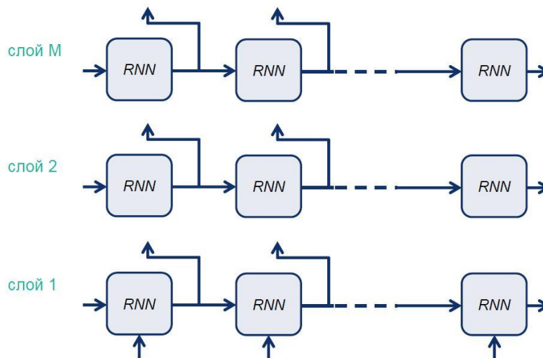
Рис. 48 Схема многослойной рекуррентной нейронной сети развернутой во времени
