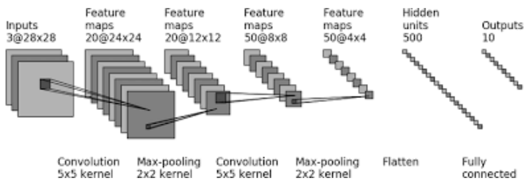
Рис. 67 Сверточная нейронная сеть
