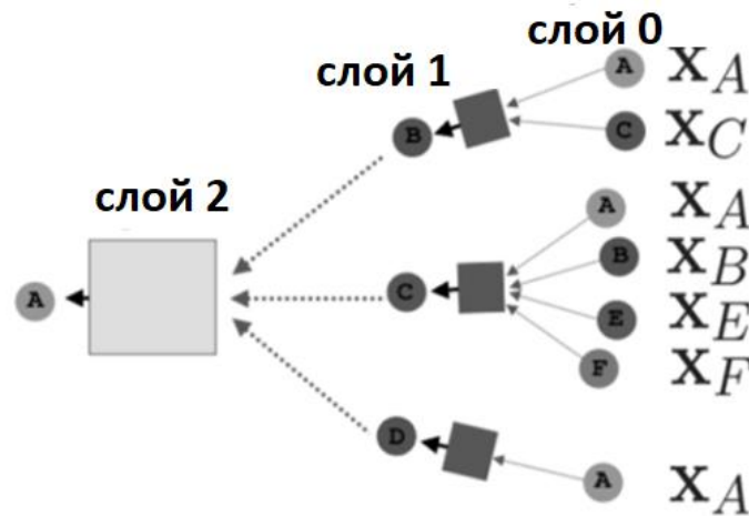
Рис. 83 Многослойная графковая нейронная сеть
