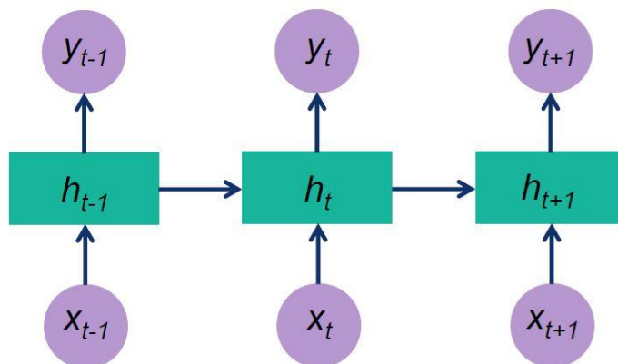
Рис. 47 Схема рекуррентной нейронной сети развернутой во времени
