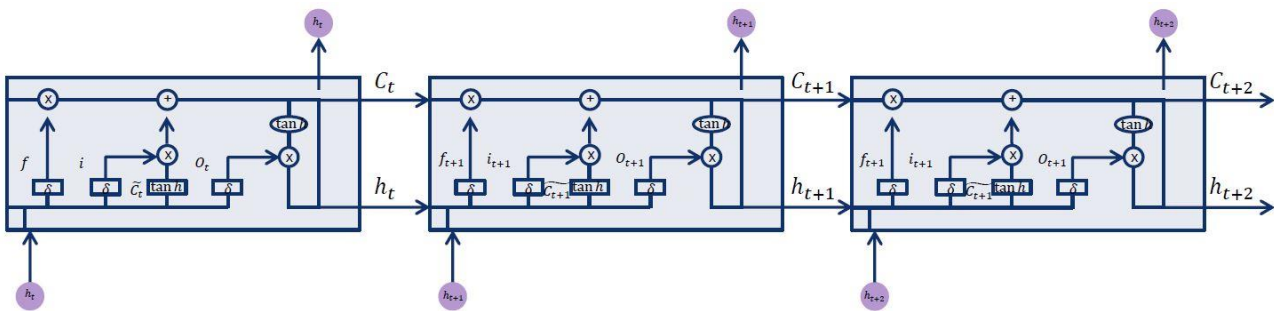
Рис. 50 Схема LSTM нейронной сети
