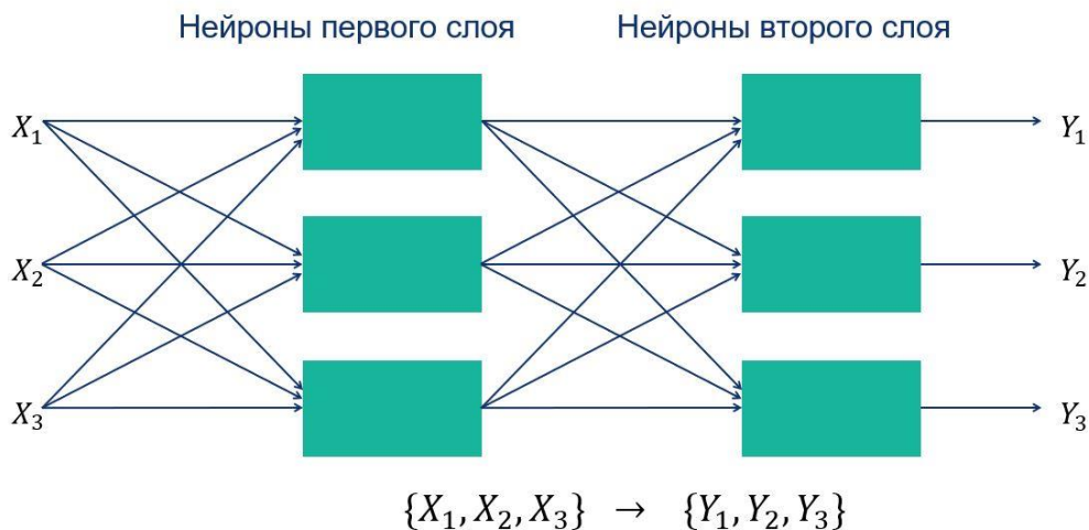
Рис.31 Многослойные нейронные сети
