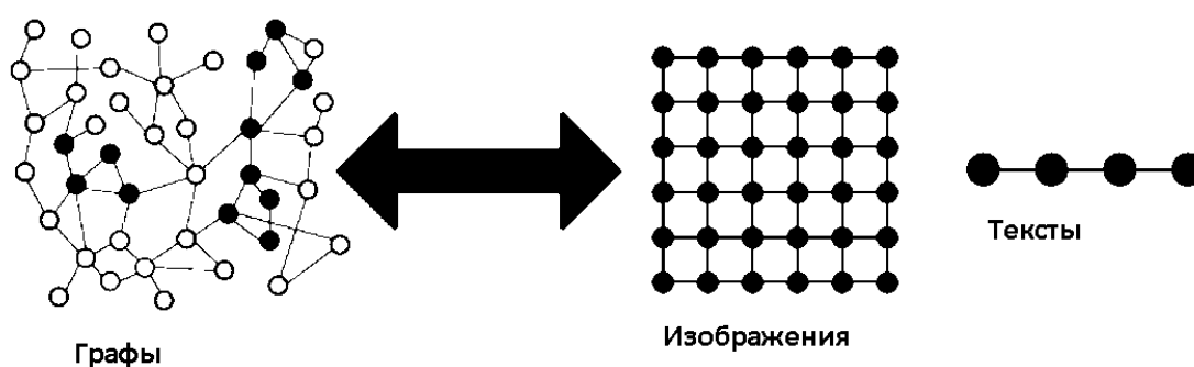
Рис. 80 Представление различных видов данных в виде графов.
