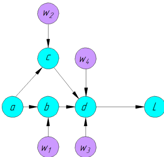
Рис.9 Визуализация вычислительного графа
