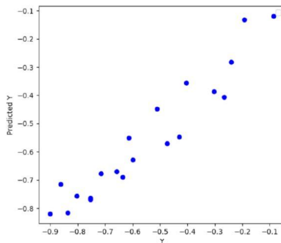
Диаграмма рассеяния
