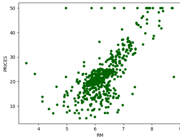
Рис. 38 Зависимость цены дома от количества комнат
