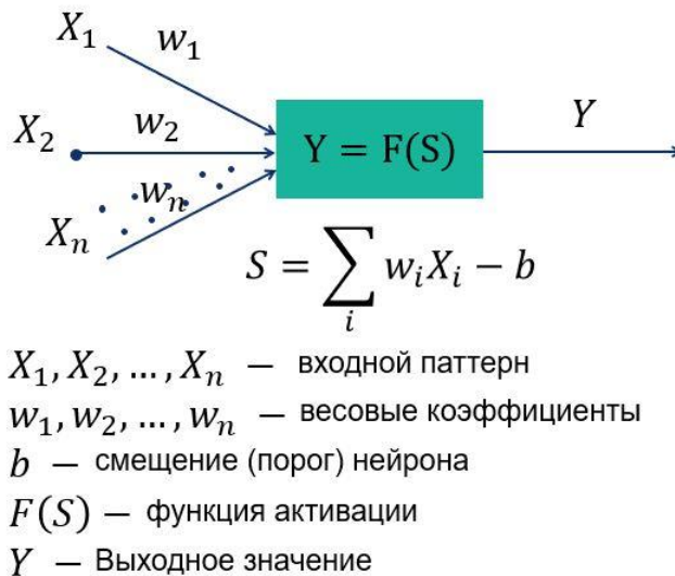
Рис. 24 Формальный нейрон
