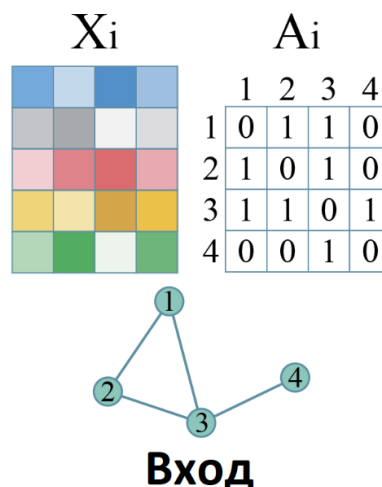
Рис. 79 Матрица смежности
