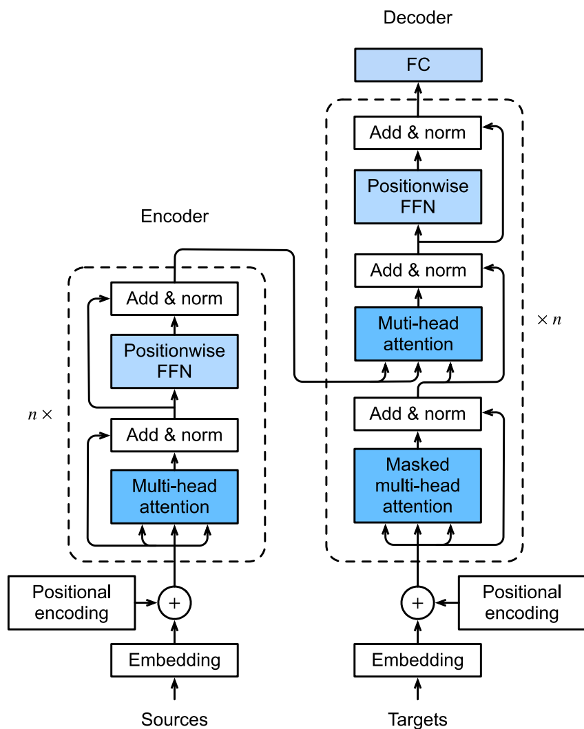
Рис. 89 Архитектура трансформера
