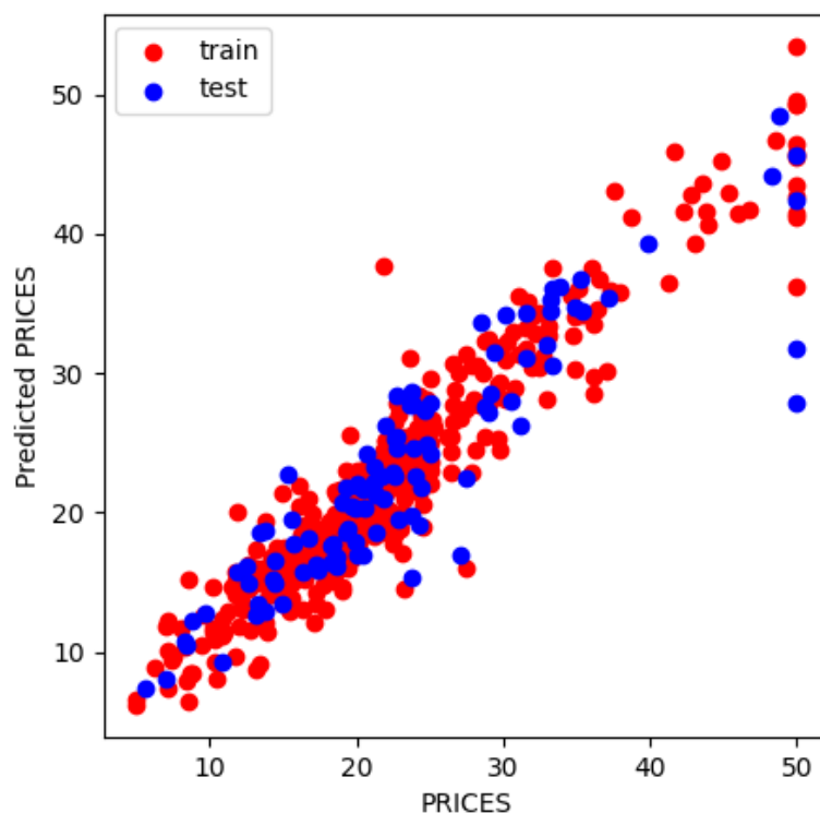
Рис. 45 Диаграмма рассеяния
