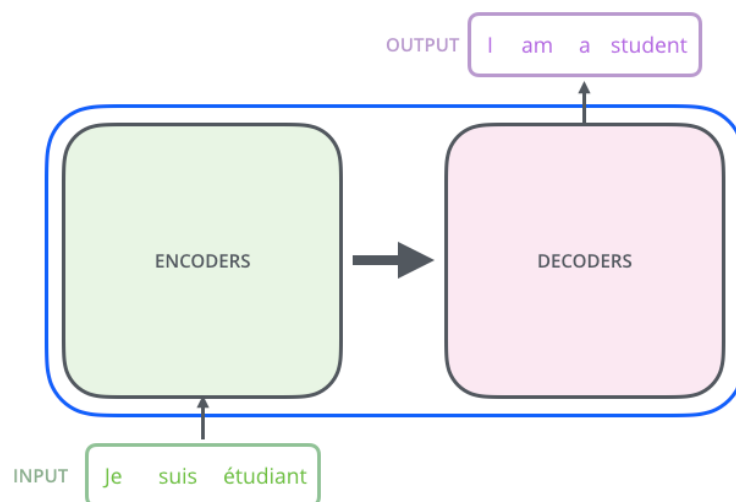
Рис. 87 Архитектура Encoder -decoder
