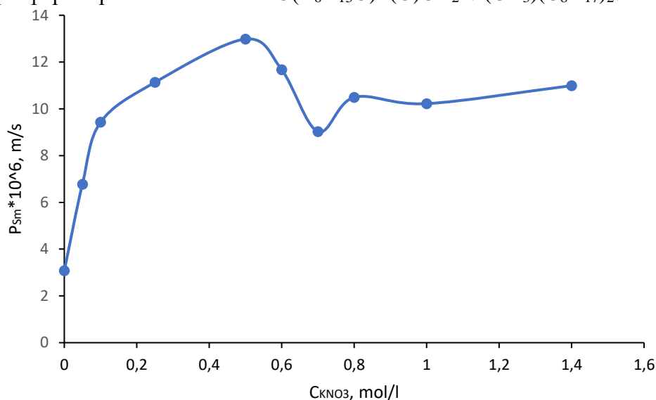
Рисунок 1. График зависимости проницаемости P_{\text{Sm}} от концентрации C_{\text{KNO}_3}
