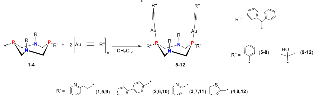
Схема 1. Синтез комплексов золота (I) 5-12.
