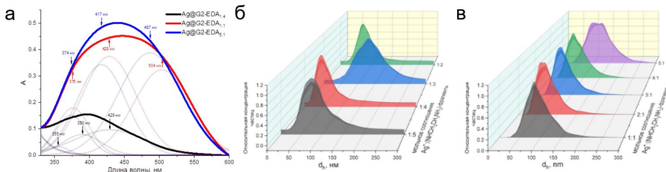
Рисунок 1. Электронные спектры поглощения образцов Ag@G2-EDA 1.4 , 1.1, 5.1 (а) и данные NTA-анализа образцов Ag@G2-EDA 1.4-1.2 (б), и Ag@G2-EDA 1.1-5.1 (в) при T_{\text{синт.}} = 50^{\circ}\text{C} .
