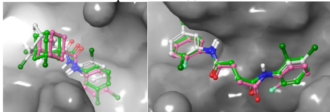
Рисунок 1. Суперимпозиция потенциальных ингибиторов в tBRCT домене белка BRCA1 .
