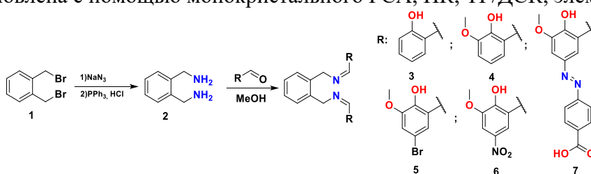
Рисунок 1. Схема получения целевых оснований Шиффа на основе o -ксилилендиамина 3-7 .
