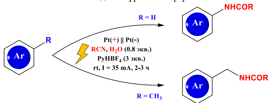
Рисунок 1. Электрохимический синтез N -фениламидов и N -бензиламидов
