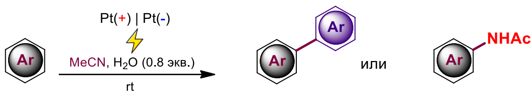
Рисунок 1. Получение биарилов и N -фениламинов в условиях электроокисления.
