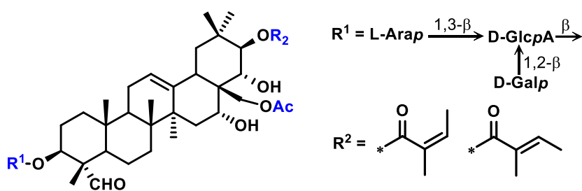
Рисунок 1. Структура полемониозидов.
