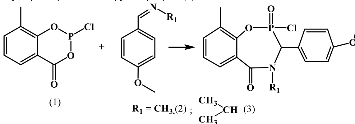
Схема 1. Схема взаимодействия хлорфосфита (1) с имидами (2,3)
