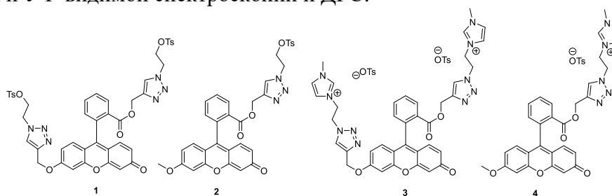
Рисунок 1. Структуры синтезированных соединений 1-4 .
