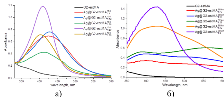
Рисунок 1. Данные УФ-Вид спектроскопии образцов \text{Ag}@G2\text{-estMA}_{1:70-1:4}^{100} ( T = 100^{\circ}\text{C} ) (а) и образцов \text{Ag}@G2\text{-estMA}_{1:70-1:4}^{365\text{nm}} ( \lambda_{\text{иниц.}} = 365 \text{ nm} ) (б).
