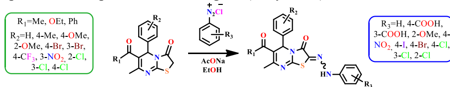
Рисунок 1. Схема синтеза 2-арилгидразонов тиазоло[3,2- a ]пиримидина [3]
