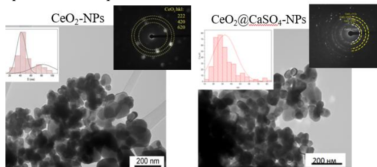
Рисунок 1. Характеристики \text{CeO}_2 -NPs и \text{CeO}_2@\text{CaSO}_4 -NPs по результатам ПЭМ и ED-анализа.
