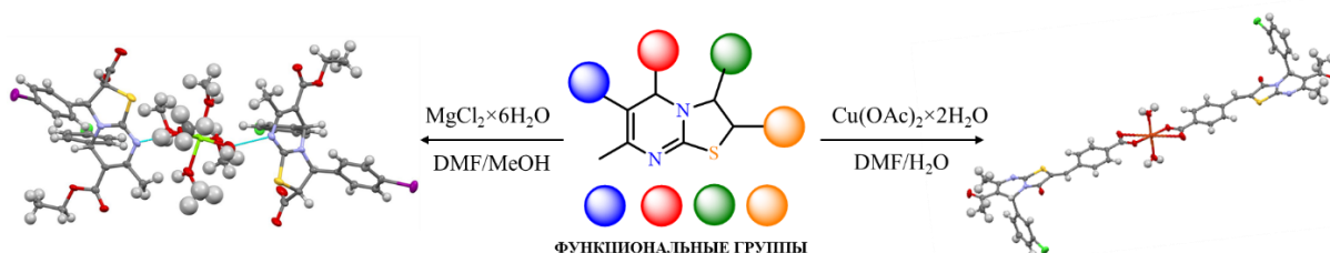
Рисунок 1. Схема получения металлокомплексов на основе производных тиазоло[3,2- a ]пиримидина.
