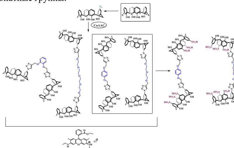
Рисунок 1. Синтез азид-производного каликс[4]арена и получение бискаликсаренов.
