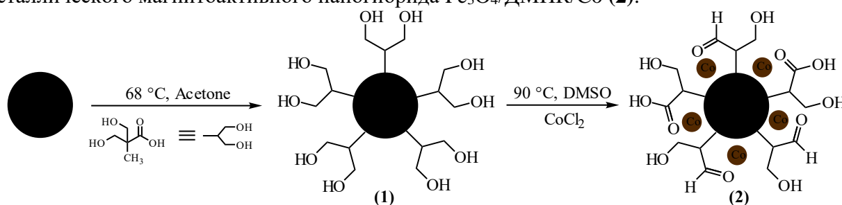
Рисунок 1. Схема синтеза наноггибридов \text{Fe}_3\text{O}_4/\text{ДМПК}/\text{Co} .
