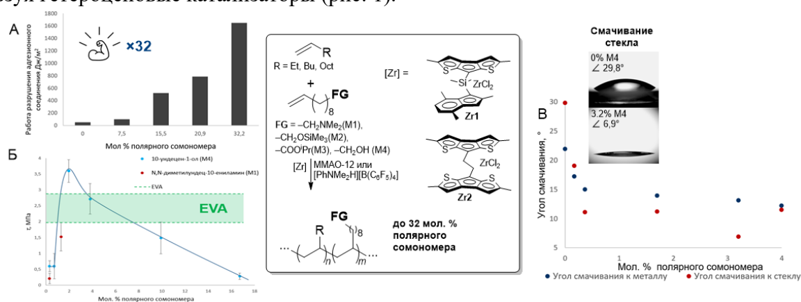
Рисунок 1. А. Значения работы разрыва адгезионного соединения для сополимеров гексена-1 с М4. Б. График зависимости напряжения разрыва адгезионного соединения для сополимеров бутена-1 с М1 и М4. В. Углы смачивания для сополимеров децена-1 с М4.
