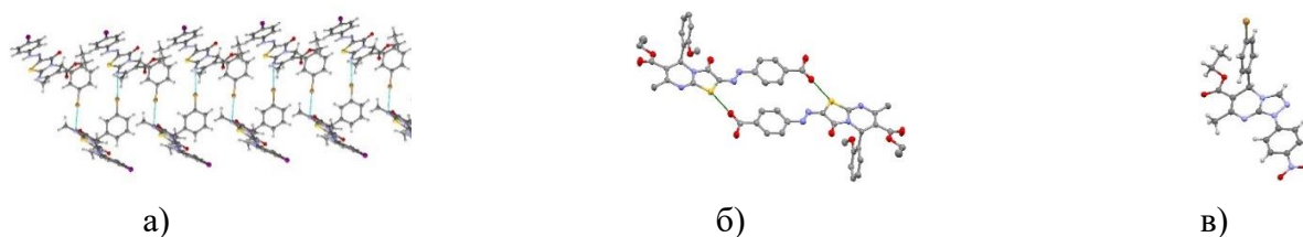
Рисунок 2. а) Геометрия и б) гомохиральные цепочки, в) халькогенно-связанные димеры 2-арилгидразонов тиазоло[3,2- a ]пиримидина в кристаллической фазе
