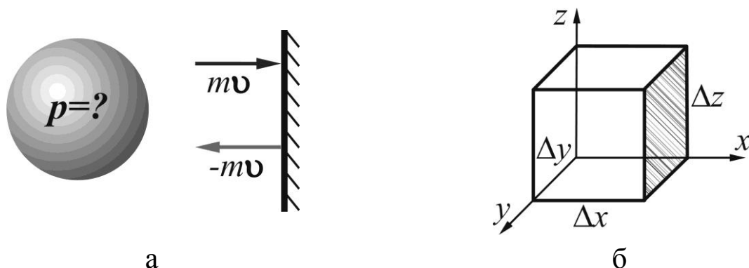
Рис. 4.6. а) – Схематическое представление изменения импульса частицы m\mathbf{v} при отскоке от стенки сосуда, б) – иллюстрация модели для расчёта давления на стенку элементарного куба – грань площадью \Delta S = \Delta z \cdot \Delta y (заштрихована)
