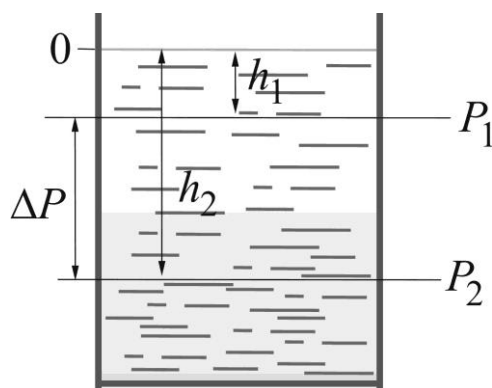
Рис. 2.2. Давление в покоящейся жидкости
