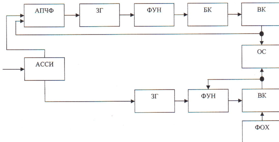
Рис. 6. Структурная схема развёртки
