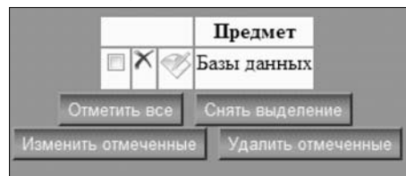
Рис. 20. Список предметов
