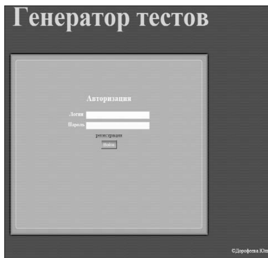
Рис. 1. Форма авторизации
