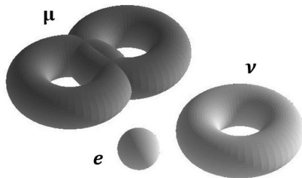
Рис.: 14. Простейшие структуры - лептоны
