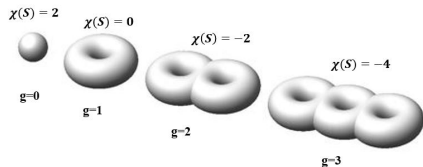
Рис.: 13. Классификация простейших топологических ячеек
