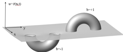
Рис.: 18. Барионы
