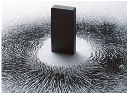
Рис.: 4. Силовые линии магнитного поля
