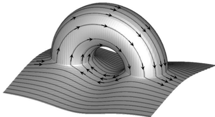
Рис.: 5. Ручка Уилера и “заряд без заряда”
