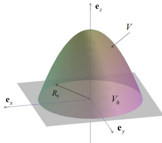
Рис.: 21. Отличие объемов интегрирования
