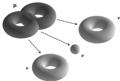
Рис.: 16. Топологическая реконструкция распада \mu -она
