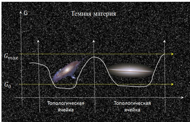
Рис.: 22. Темная материя \equiv эффективная гравитационная постоянная
