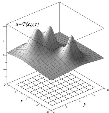
Рис.: 8. Физическая гиперповерхность и функция высоты
