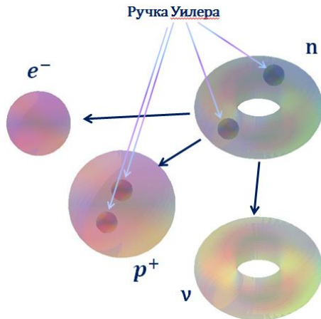
Рис.: 19. Реконструкция распада нейтрона
