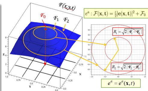
Рис.: 10. Функция высоты - квадрат расстояния в пространстве маркеров
