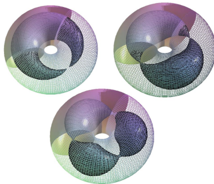
Рис.: 17. Три типа нейтрино
