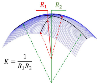
Рис.: 6. Гауссова (внешняя) кривизна
