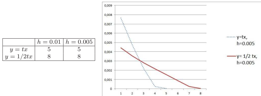
Рис. 3. Число итераций для достижения точности \varepsilon = 0.0001 при y_d = t \sin(\pi x) , итерационном параметре \rho = 1 и различных ограничениях y_{\max} \equiv y . На графике приведено поведение нормы невязки \|v\|_{D^{-1}} .
