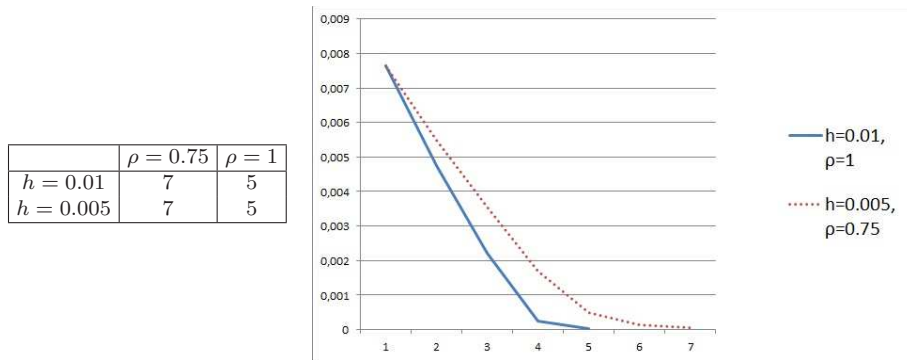
Рис. 1. Число итераций для достижения точности \varepsilon = 0.0001 при y_d = t \sin(\pi x) и ограничении y_{\max} = tx . На графике приведено поведение нормы невязки \|v\|_{D^{-1}} для различных параметров
