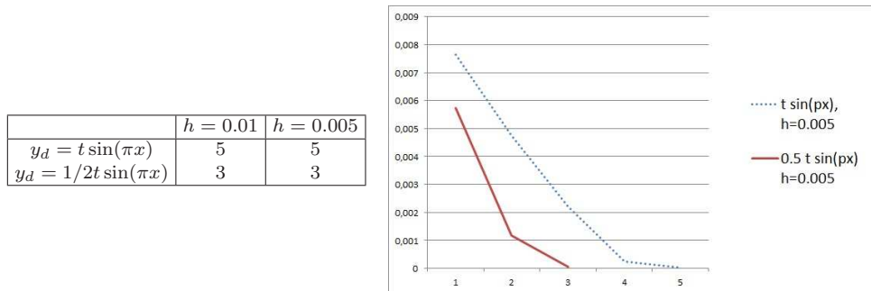
Рис. 2. Число итераций для достижения точности \varepsilon = 0.0001 при ограничении y_{\max} = tx , итерационном параметре \rho = 1 для различных y_d . На графике приведено поведение нормы невязки \|v\|_{D^{-1}} для различных параметров
