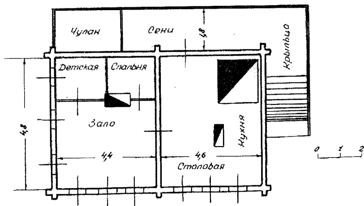
Рис. 7. Дом Семяхина С.М. постройки 1951 года (д. Иваново Ядринского района ЧАССР)
